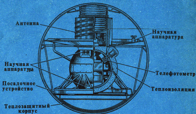
Спускаемый аппарат
