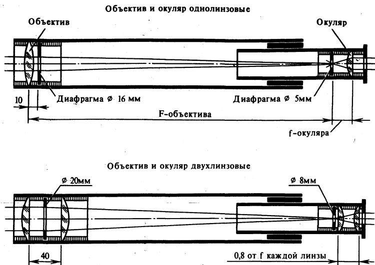
Рис. 40. Самодельный рефрактор
