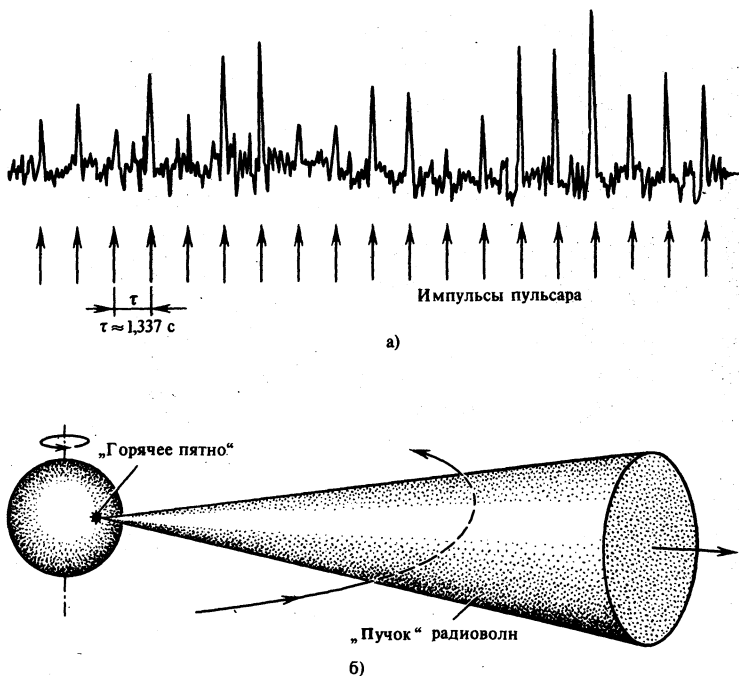
Рис. 36. Пульсар: а — пример записи радиоизлучения пульсара, б — модель пульсара.
