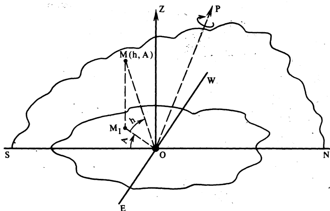
Рис. 42. Горизонтальные координаты
