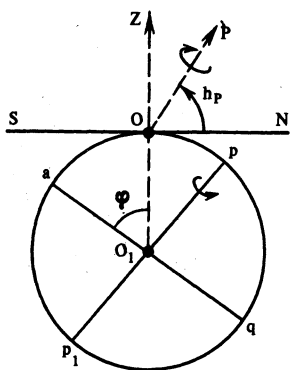
Рис. 43. Теорема о высоте полюса мира
