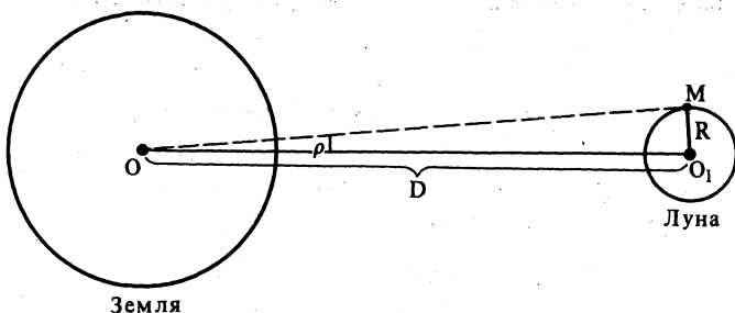
Рис. 7. Определение размеров небесных тел Солнечной системы
