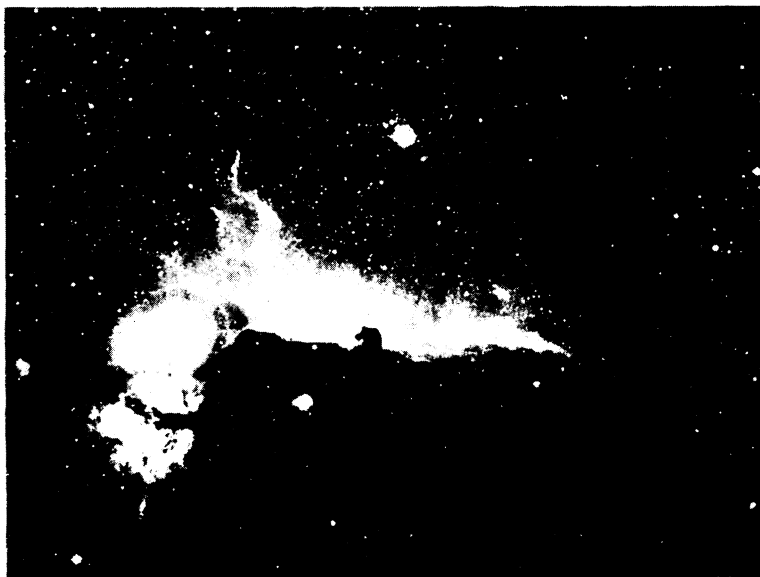
Рис. 52. Темная туманность «Конская Голова» (созвездие Ориона)
