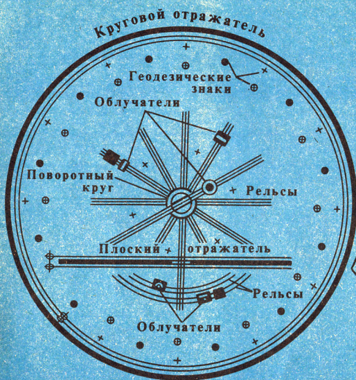
Схема размещения основных частей радиотелескопа
