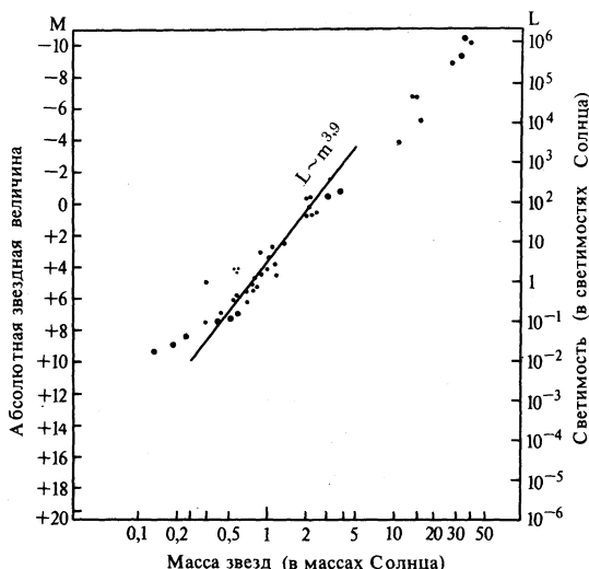
Рис. 55. Диаграмма «масса — светимость»
