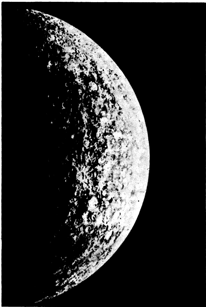
Рис. 15. Вид Меркурия с близкого расстояния («Маринер-10») Поверхность какого небесного тела вам напоминает поверхность Меркурия?
