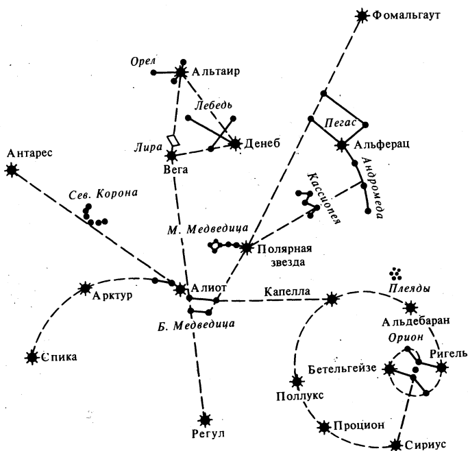
Рис. 41. Взаимное расположение ярких звезд
