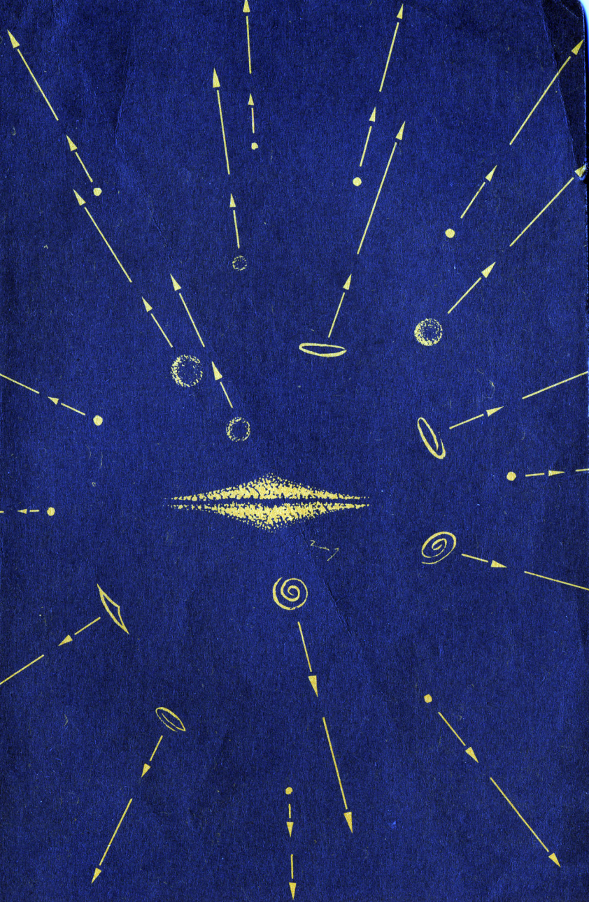
Расширяющаяся Метагалактика
