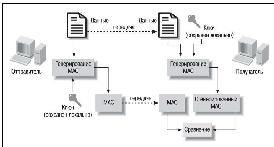
Рис. 4.9. Использование кода аутентификации сообщения ( Message Authentication Code )
