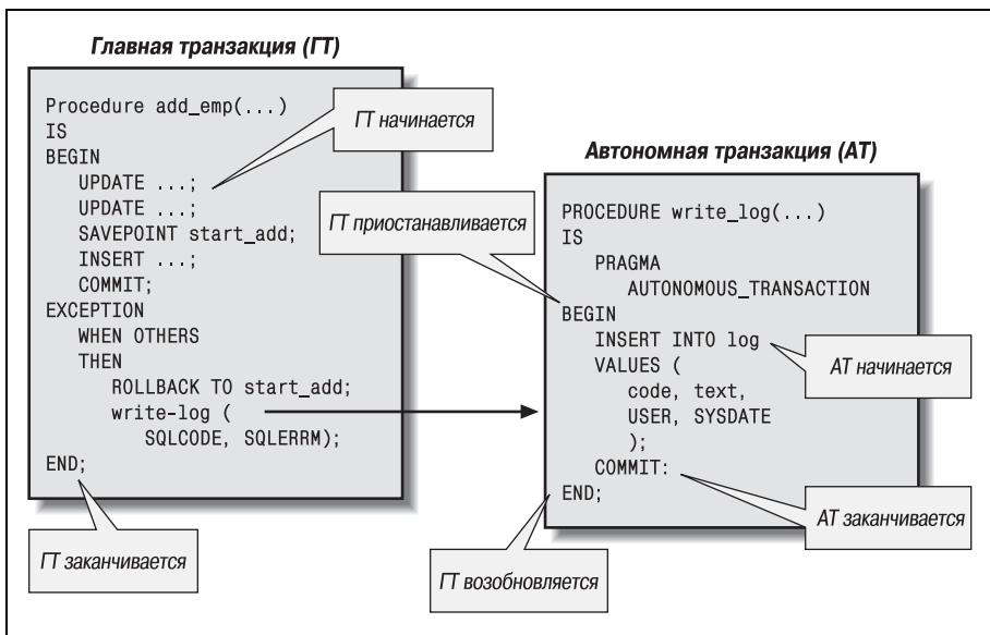
Рис. 1.5. Передача управления между главной и автономной транзакциями
