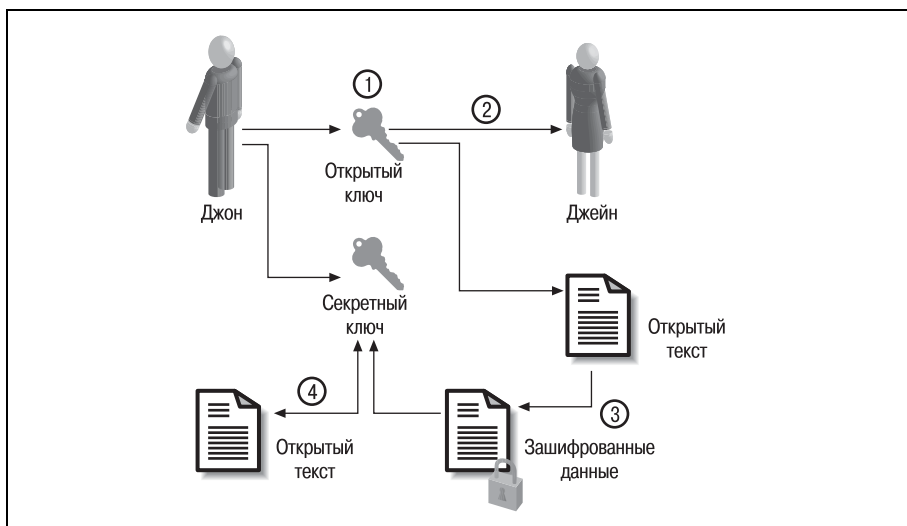
Рис. 4.2. Базовая схема асимметричного шифрования
