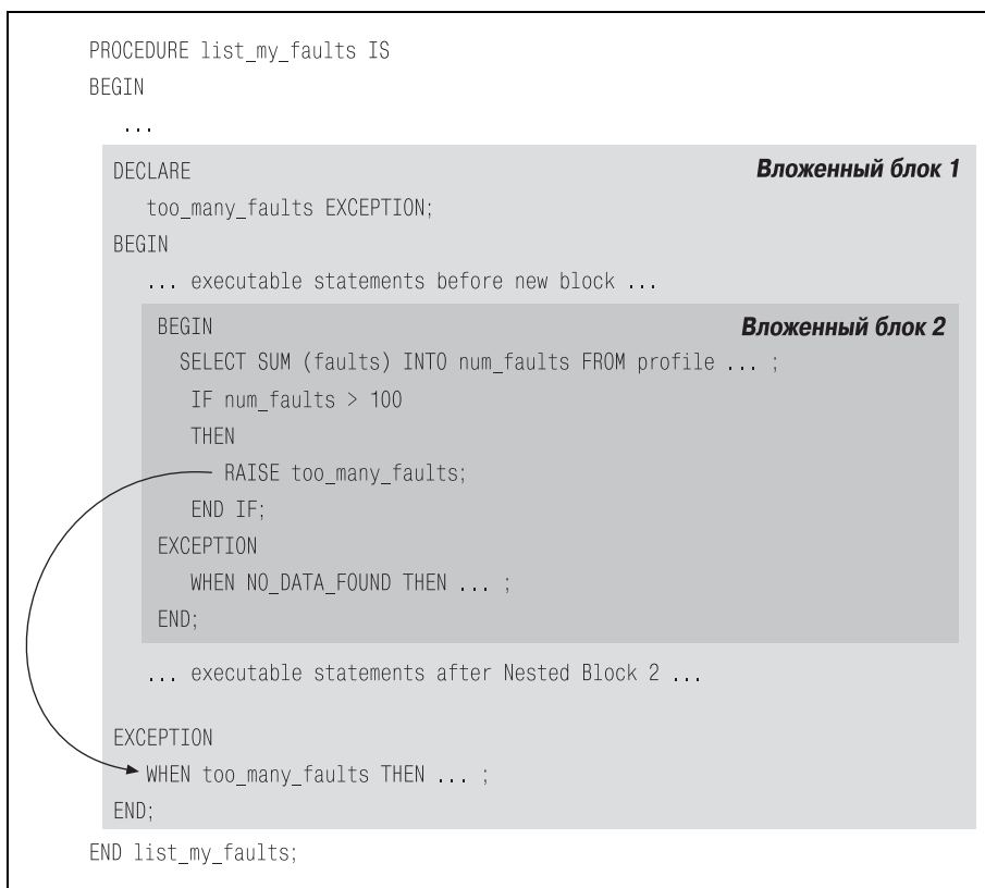
Рис. 1.3. Передача необработанного исключения
