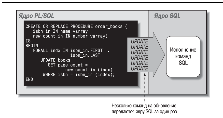
Рис. 1.4. Одно переключение контекста в операторе FORALL
