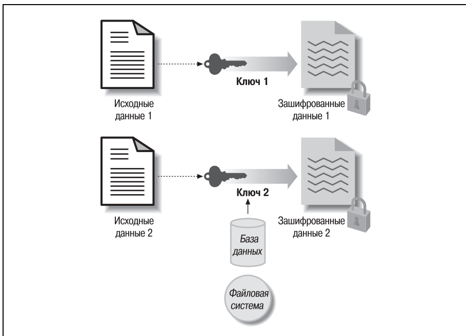
Рис. 4.4. Использование нового ключа для каждой строки
