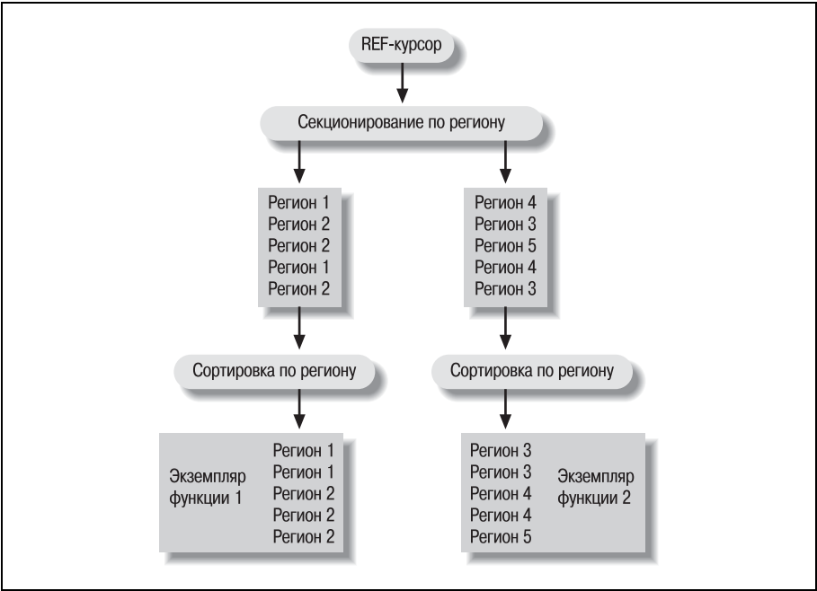
Рис. 3.2. Распараллеленная табличная функция, секционированная и отсортированная по региону
