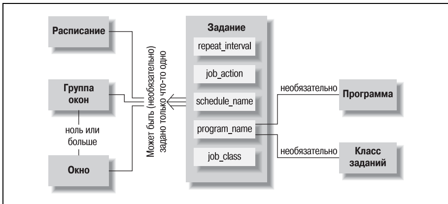
Рис. 8.1. Составляющие планировщика Oracle
