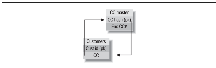
Рис. 4.10. Хранение зашифрованной информации о кредитных картах
