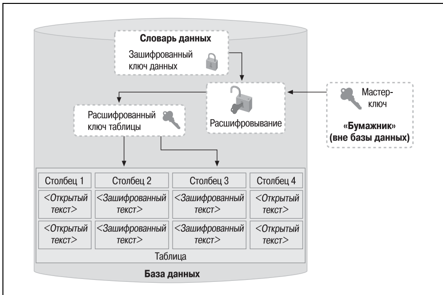
Рис. 4.7. Модель прозрачного шифрования данных
