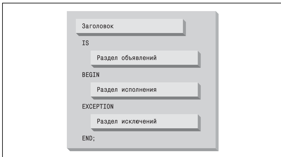
Рис. 1.1. Структура блока PL/SQL
