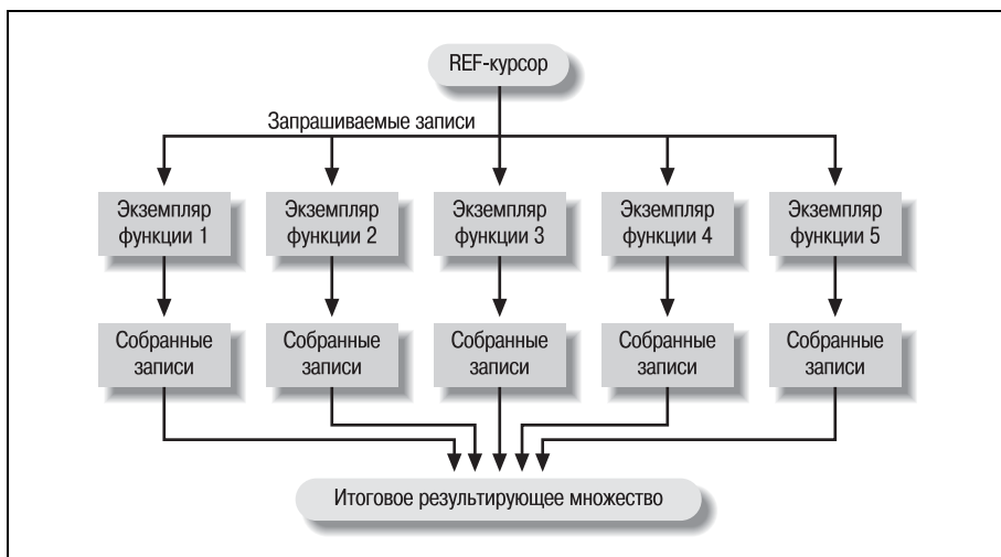
Рис. 3.1. Распараллеленная табличная функция
