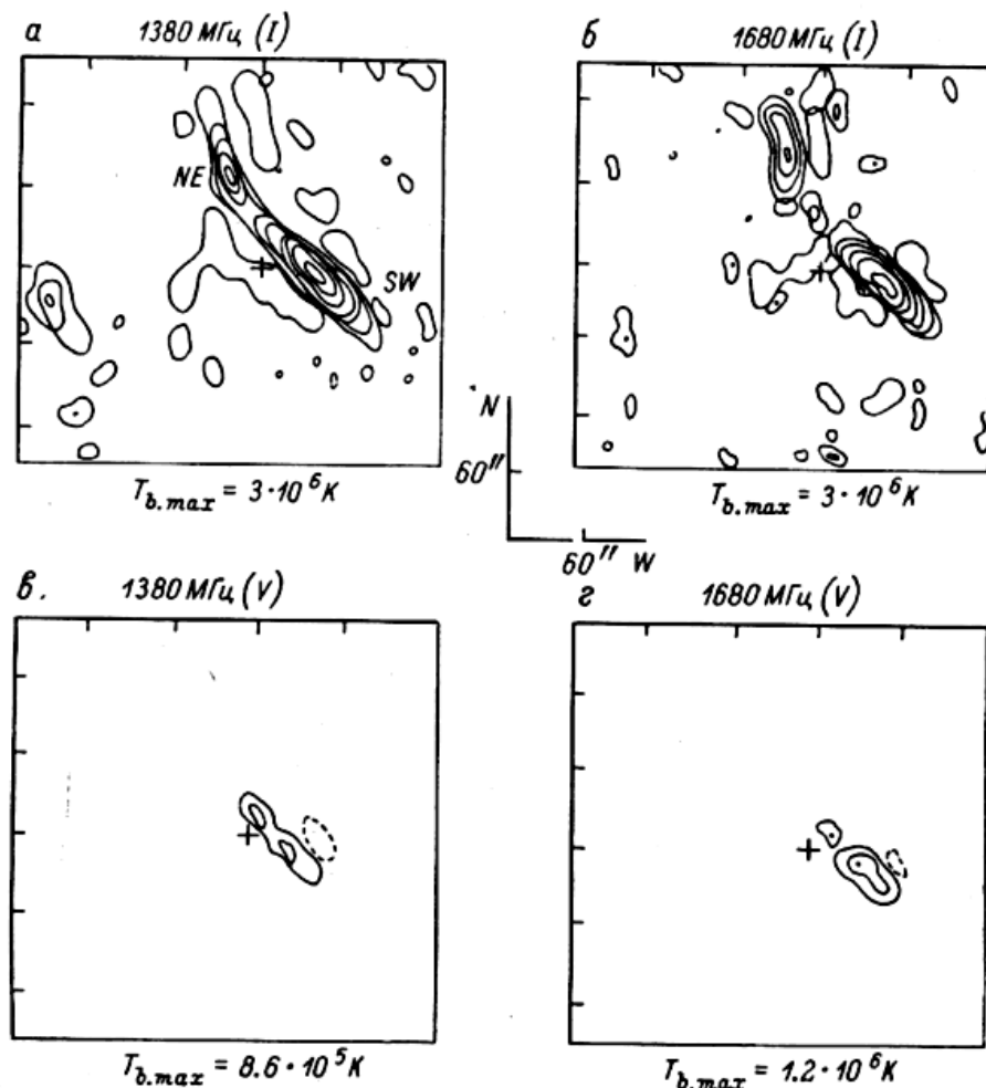
Рис. 8. Синтезированные на VLA радиокарты участка активной области AR3804. Координаты креста на 13 h UT: N13E35. Контуры на картах интенсивности (I) соответствуют уровням 0.2, 0.3, ..., 0.9 от T_{b, \max} .
