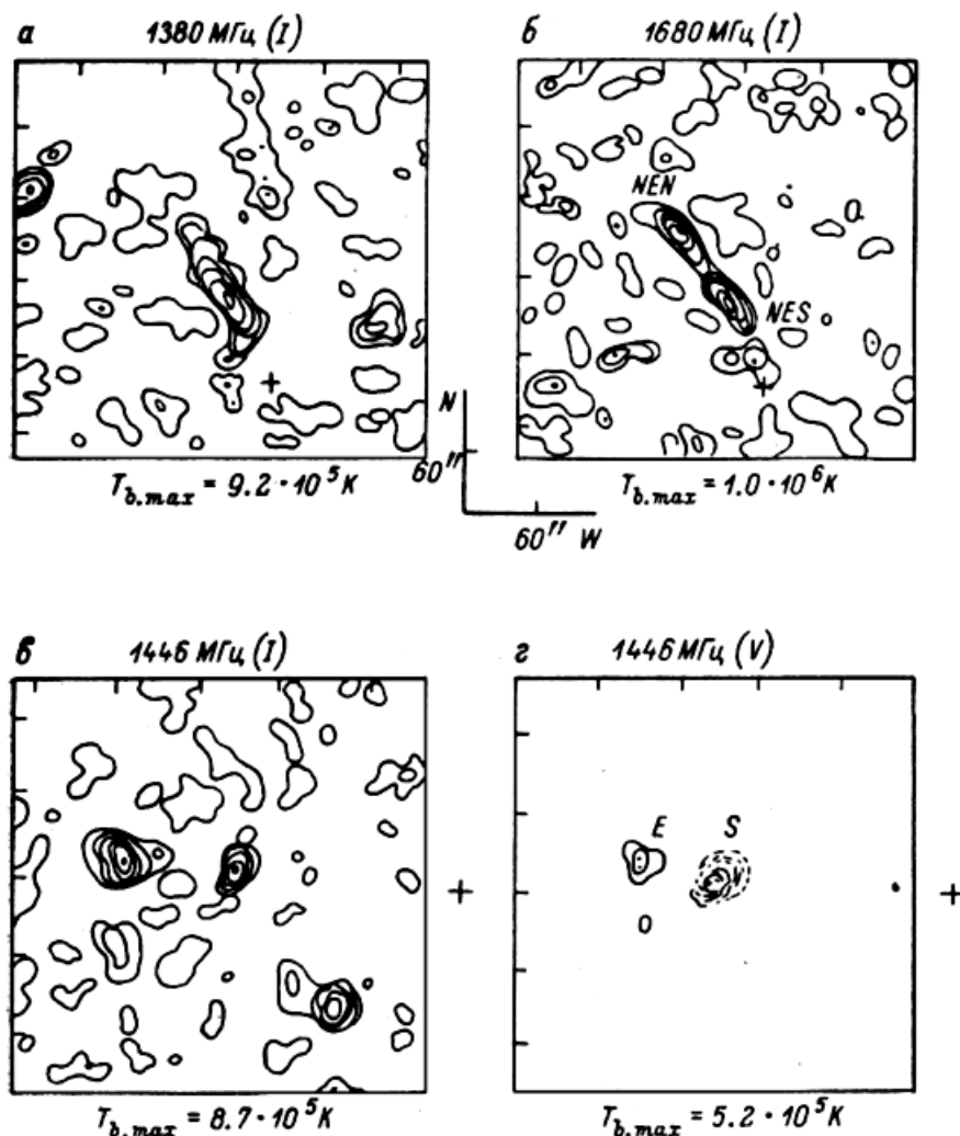
Рис. 9. Синтезированные на VLA радиокарты участков активных областей AR3804 и AR3826. Координаты крестов на 13 h UT: N13 E21 на 13.07.82 (AR 3804) и S15E4.5 на 27.07.82 (AR 3826).
