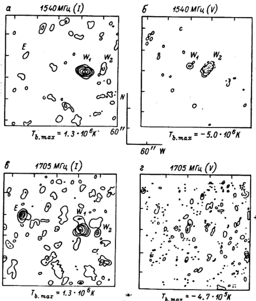
Рис. 11. Синтезированные на VLA радиокарты участка активной области AR3826. Координаты креста на 13 h UT: S15W8.5. Контуры на картах интенсивности (I) соответствуют уровням 0.2, 0.3, ..., 0.9 от T_{b, \max} .
