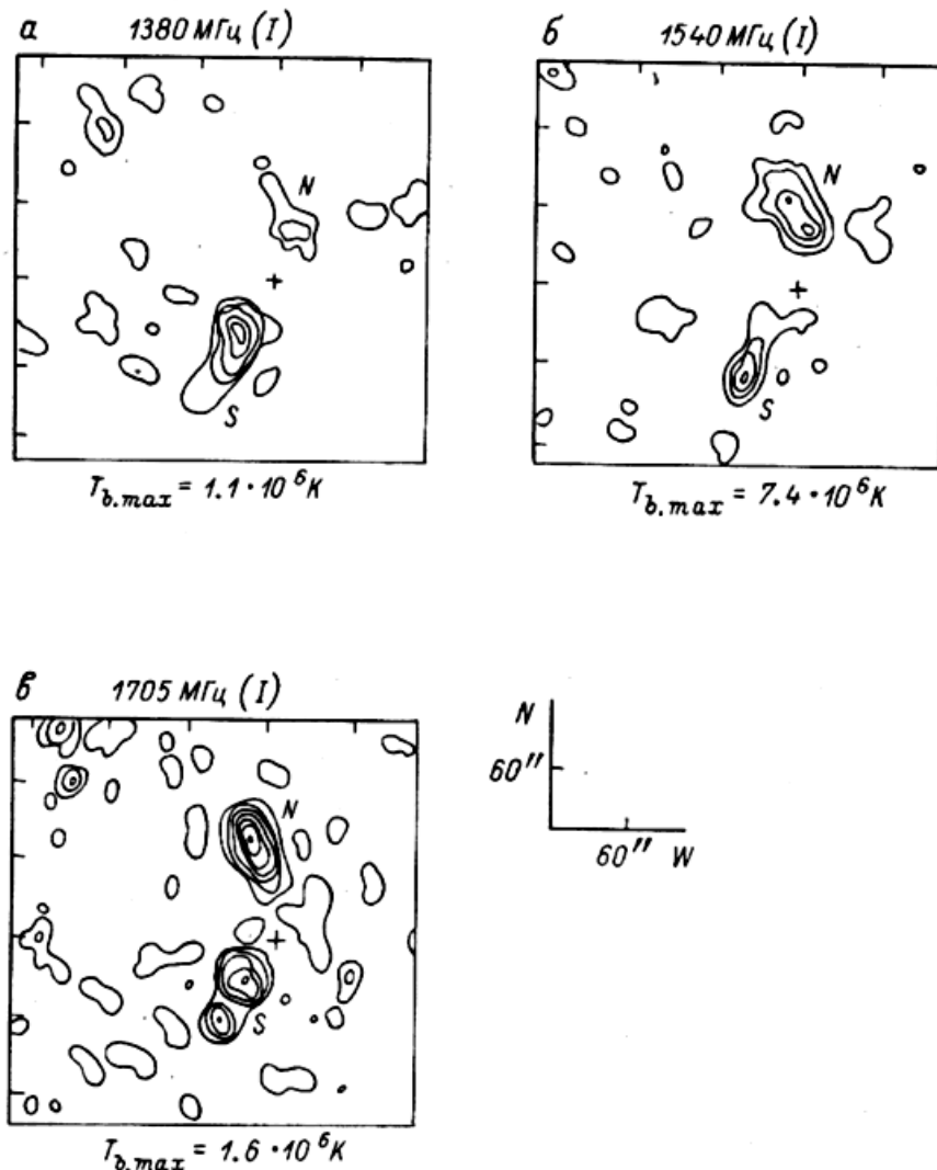
Рис. 10. Синтезированные на VLA радиокарты участка активной области AR3804. Координаты креста на 13 h UT: N09W64. Контуры на картах интенсивности ( I ) соответствуют уровням 0.2, 0.3, ..., 0.9 от T_{\text{в}, \text{max}} .
